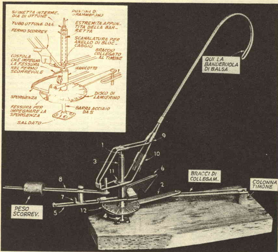
Le parti del meccanismo che sono in filo metallico possono benissimo essere realizzate con dei raggi da bicicletta, che possono ottenersi gratis da qualsiasi meccanico del ramo
